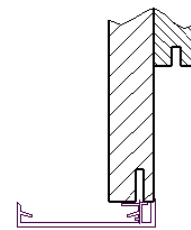
Abdeckleiste Kunststoff
