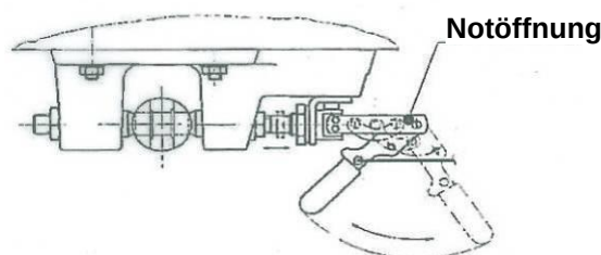
Ansicht X
