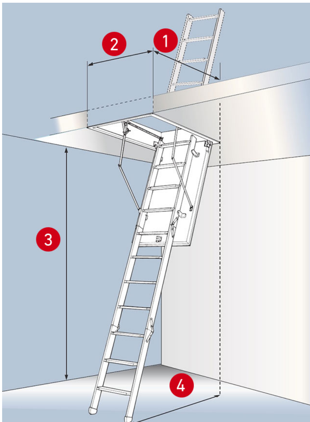
Bodentreppe clickFIX® vario | Standardmaße (Deckenöffnung)
